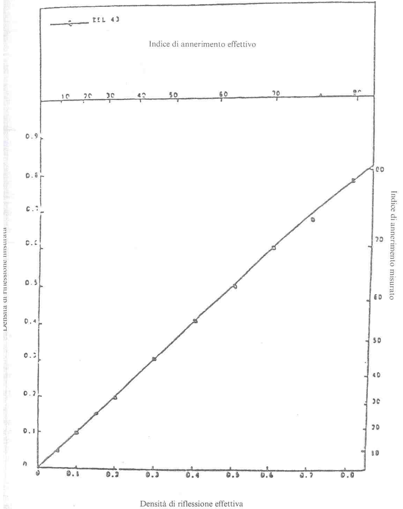
Fig. 3. Risposta del riflettometro (appendice 12, punto 2.7).
